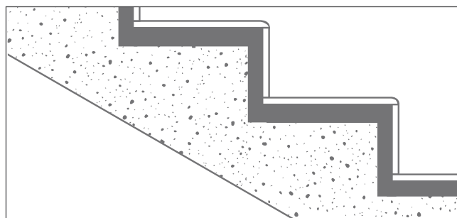
PELDAÑO CON RANURAS STEP TREAD (FLAT) WITH GROOVES
